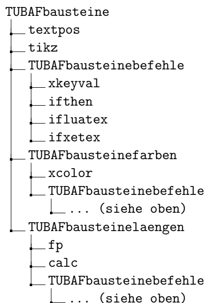
Abb. 1: Eine kurze Skizze der Paketabhängigkeiten
